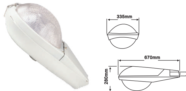
PHFR-250A 250W E40
