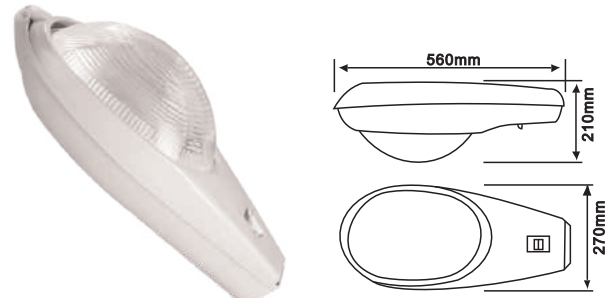
PHFR-150B E27 150W
