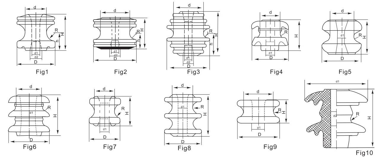
主要尺寸和性能 MAIN DIMENSIONS AND STANDARD PARTICULARS
